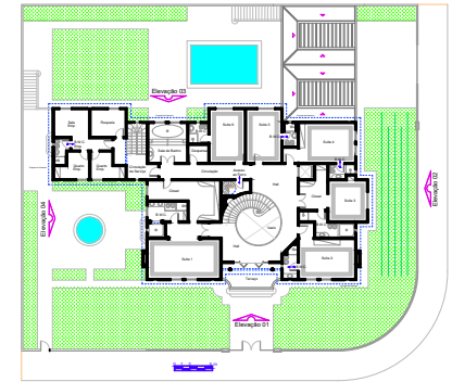
Superior A = 392,63 m 2
